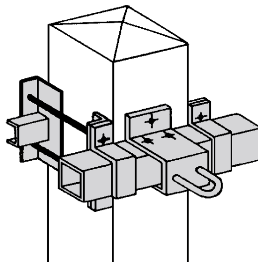
Accrochage unifilaire simple KTUNX
